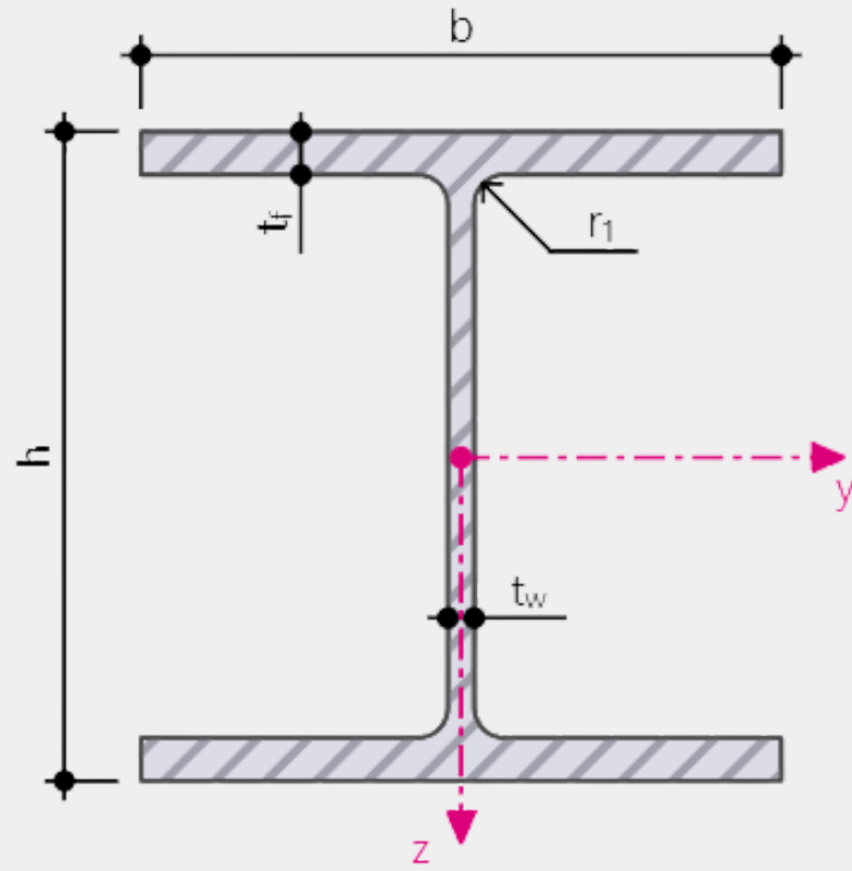
H Profil (100-1000) (HEA - HEB - HEM)
