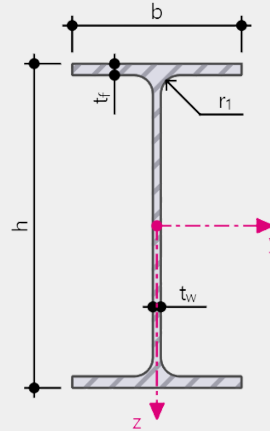
IPE Profil (80-750)
