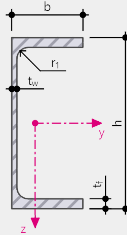
UPE Profil (80-400)
