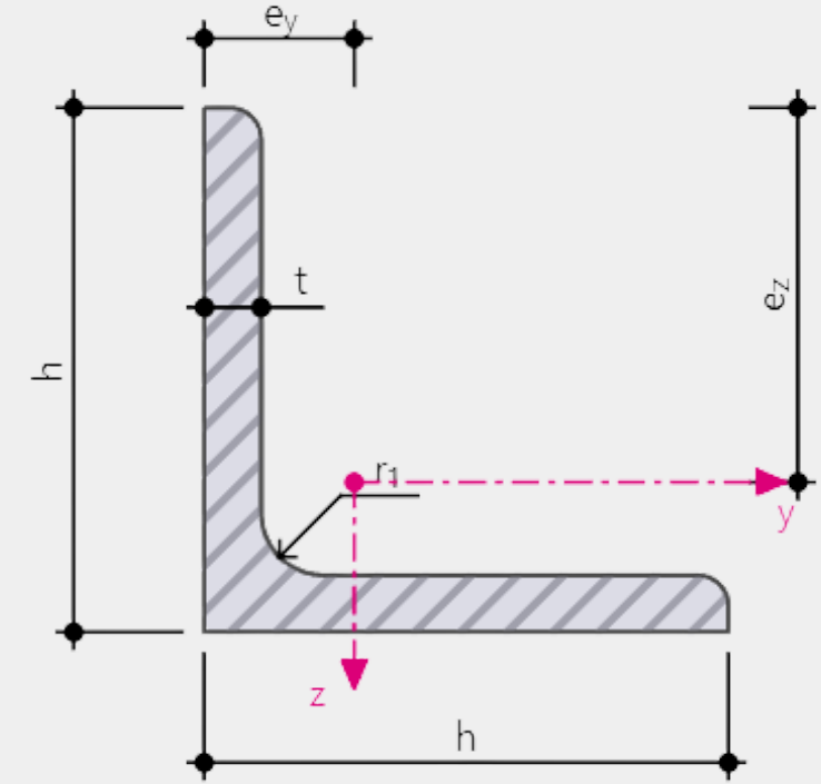
Köşebent (25-300)
