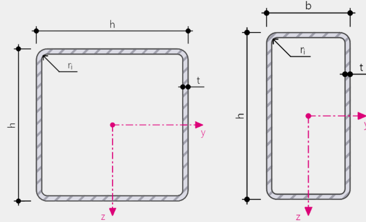
Konstrüksiyon Profiller (10*10mm & 400*400mm)
