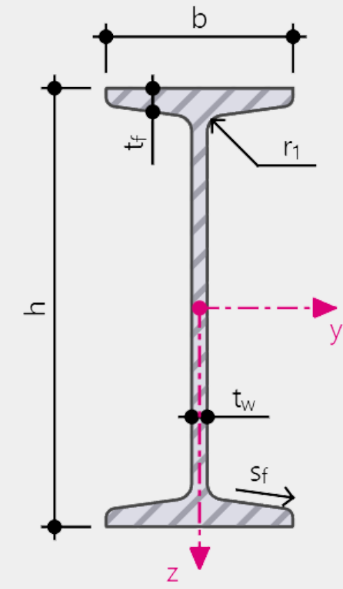
IPN Profil (80-600)
