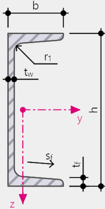
UPN Profil (40-400)
